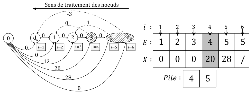
Figure 2.45: Algorithme après le traitement du sommet 3
