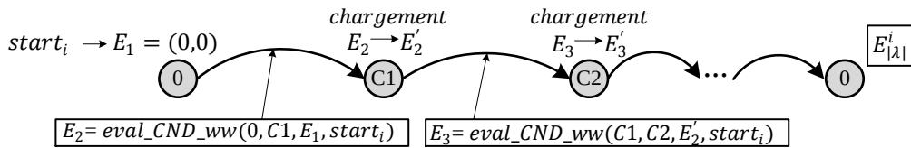
Figure 3.50: Evaluation d'un \lambda en autorisant l'attente
