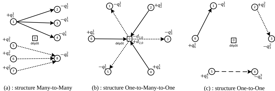
Figure 1.3 : Structures pour les GPDP
