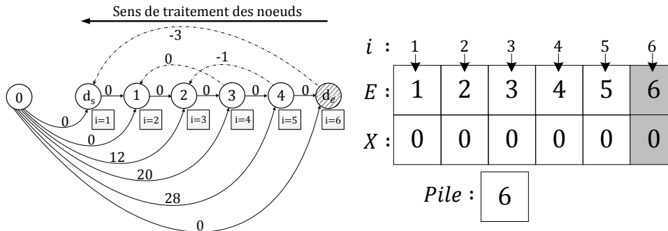
Figure 2.43: Algorithme après le traitement du sommet d_s
