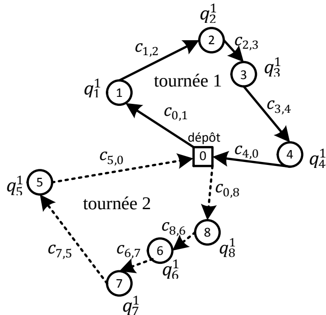
Figure 1.2 : Exemple de modélisation de GPDVRP à 8 sommets et deux véhicules
