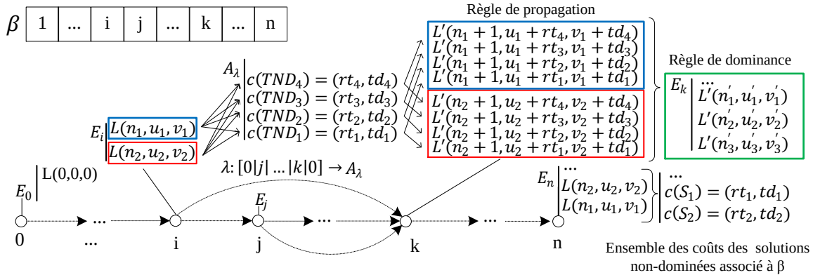
Figure 3.48: Schéma du split pour le TDVRP avec attente
