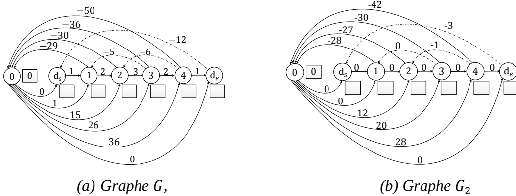
Figure 2.30: Exemple de graphe G et du graphe G_2 associé au même problème
