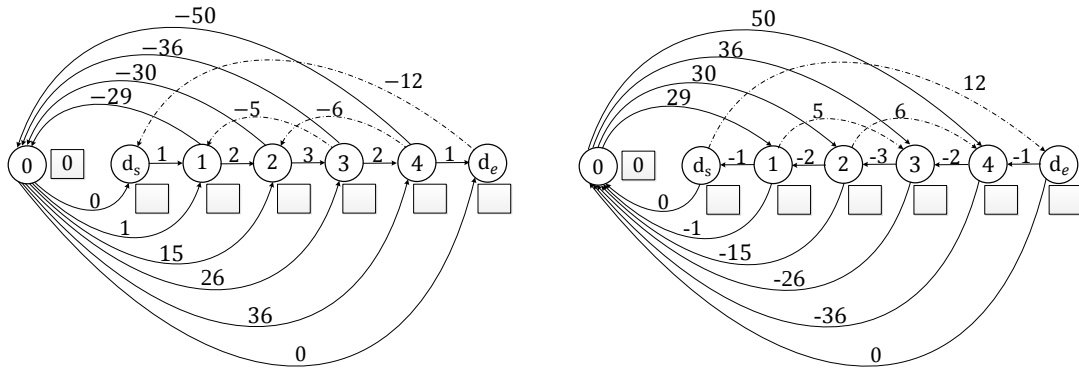
Figure 2.15: Exemple de graphes G (gauche) et G' (droite)
