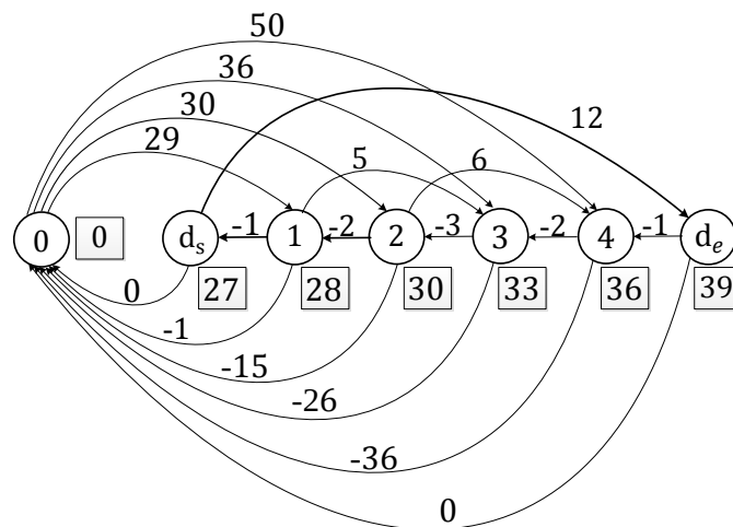
Figure 2.16: Calcul du plus court chemin en partant de 0 dans G'
