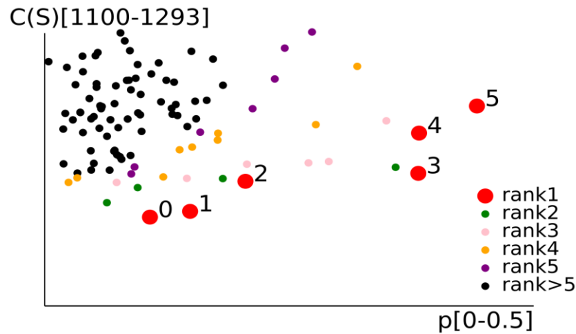
Figure 4.49 : Le tri par non-domination sur la population initiale de l'instance PR06 sous H1
