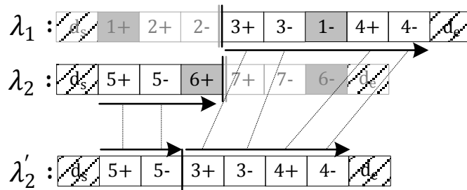
Figure 2.66 : Construction du vecteur t'_2
