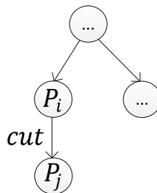
Figure 1.12 : Ajout d'une contrainte de coupe
