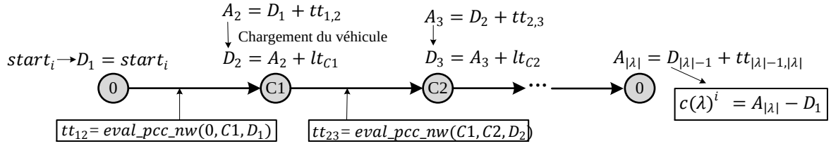
Figure 3.37: Evaluation d'un \lambda sans autoriser l'attente pour une date de départ
