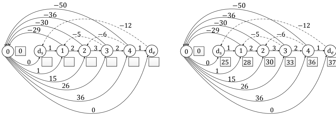
Figure 2.14: Exemple de graphe G avant et après le calcul des plus longs chemins en partant de 0
