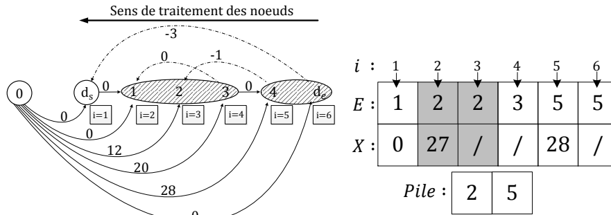
Figure 2.47: Algorithme après le traitement du sommet 1
