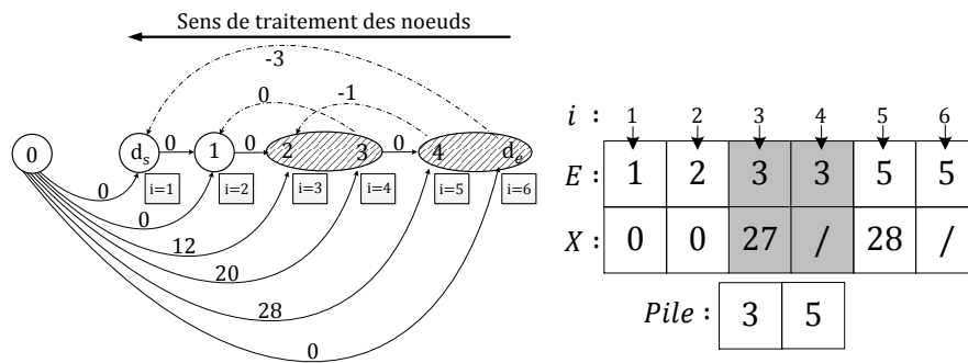
Figure 2.46: Algorithme après le traitement du sommet 2
