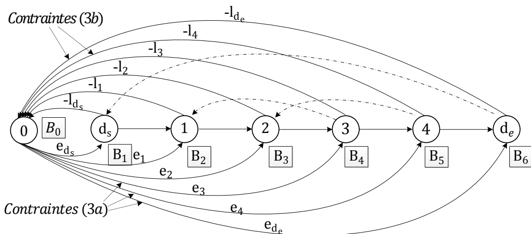
Figure 2.12: Graphe après l'ajout des contraintes (3a) et (3b)
