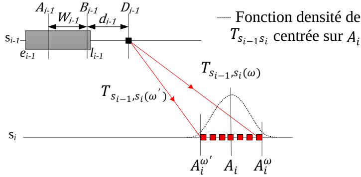
Figure 4.5 : Conséquence sur la tournée de la réalisation de T_{s_{i-1}s_i}(\omega)
