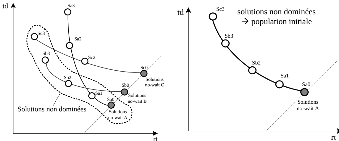
Figure 3.55 : Evaluation des \beta associés aux solutions sans attente et construction de la population initiale
