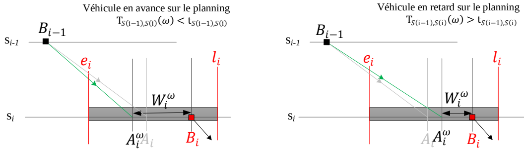
Figure 4.9 : Illustration dans le cas stochastique de l'hypothèse 1
