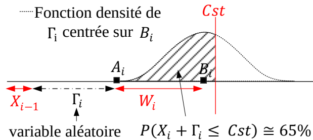
Figure 4.31 : Probabilité qu'une contrainte soit valide sous l'hypothèse 2
