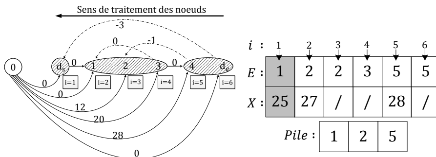
Figure 2.48: Algorithme à la fin de l'étape 2
