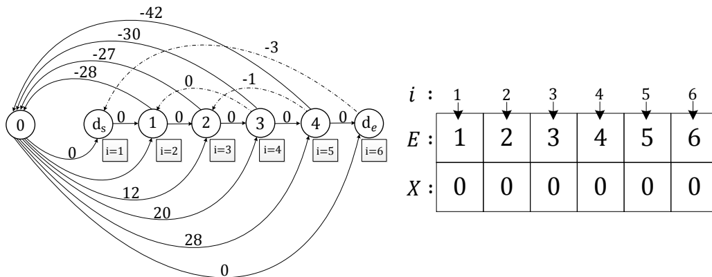
Figure 2.37: Valeur des vecteurs E et X initiaux
