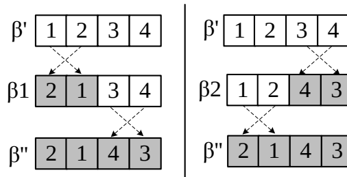
Figure 3.44 : L'ordre des permutations influence l'espace des solutions parcourut par les \beta
