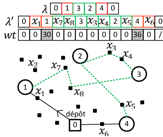
Figure 3.54: Reconstruction de la tournée si une amélioration est obtenue
