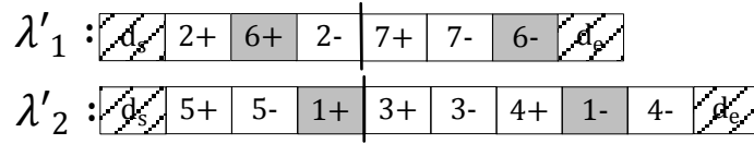
Figure 2.68 : Les vecteurs finaux obtenus
