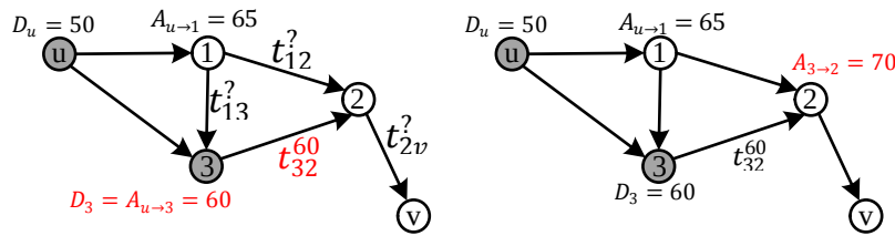
Figure 3.18 : Le sommet avec la date d'arrivée le plus tôt est propagé
