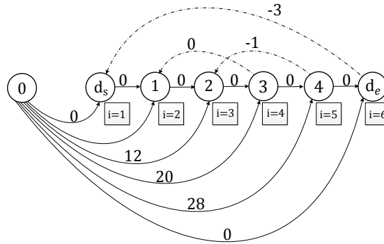
Figure 2.38: Exemple de graphe à évaluer
