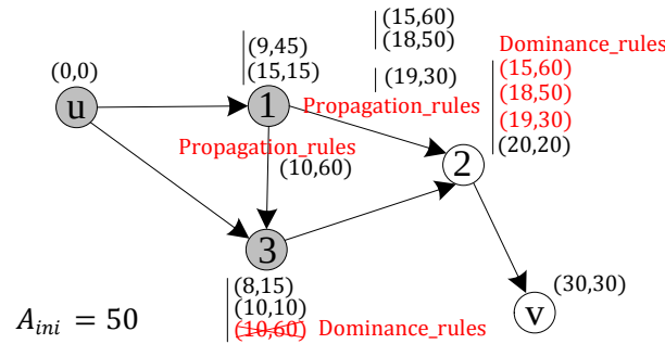
Figure 3.30 : Propagation des labels de 1 vers 2 et 3
