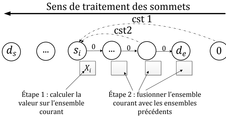
Figure 2.39: Principe de l'évaluation
