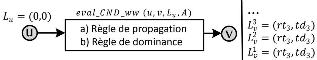
Figure 3.22 : La fonction d'évaluation associée à chaque date de début un ensemble de chemins
