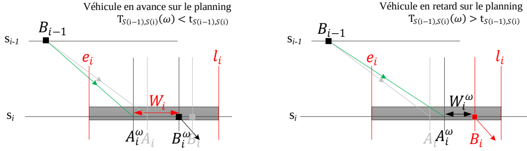
Figure 4.13 : Illustration dans le cas stochastique de l'hypothèse 3
