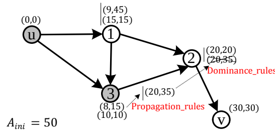
Figure 3.29 : Propagation des labels de 3 vers 2
