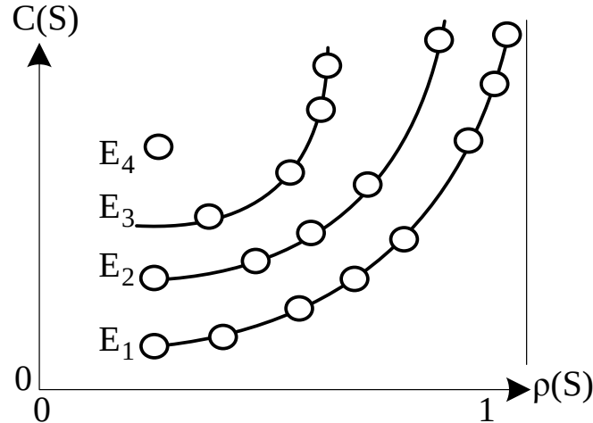
Figure 4.48 : Tri des solutions par non-domination
