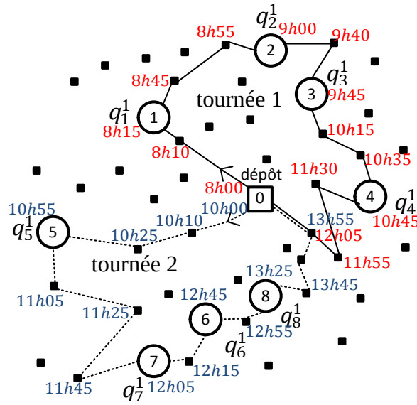
Figure 3.11 : Une solution du TDVRP à 8 sommets et deux véhicules
