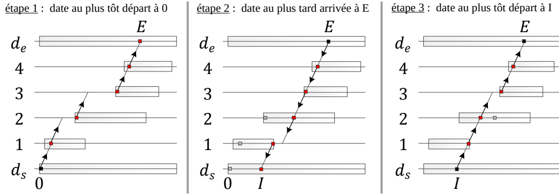
Figure 2.22: Evaluation par (Cordeau and Laporte, 2003) étape 1 à 3
