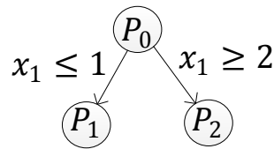
Figure 1.11 : Schémas arborescents et opération de séparation de P_0
