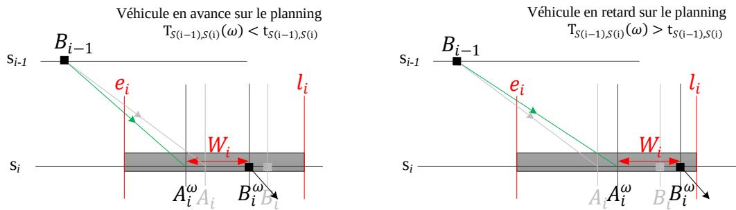
Figure 4.11 : Illustration dans le cas stochastique de l'hypothèse 2
