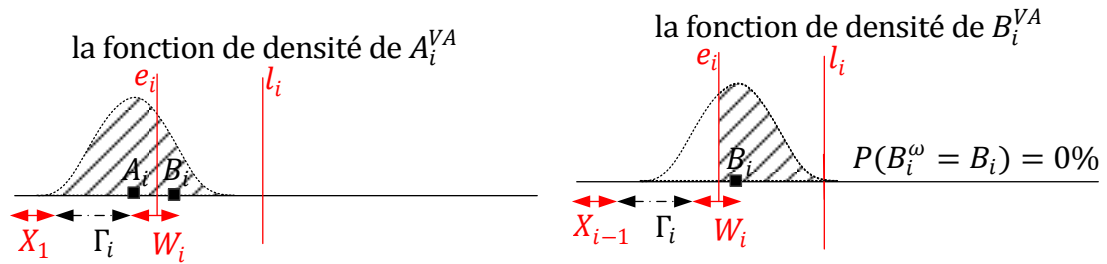
Figure 4.38 : Représentation de la loi de A_i^{VA} et B_i^{VA} sous H_2
