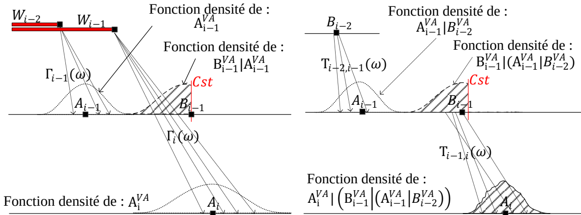
Figure 4.36 : Représentation de la loi de A_i^{VA} et B_i^{VA} sous H3
