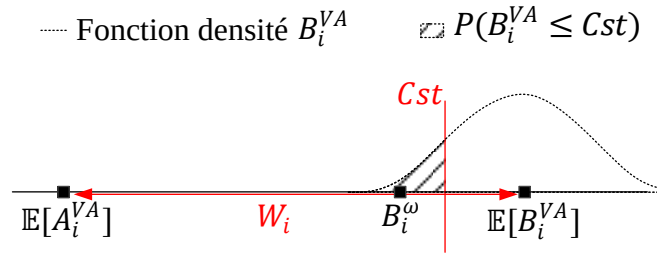
Figure 4.7 : Une contrainte non valide pour le DDARP dans le SDARP
