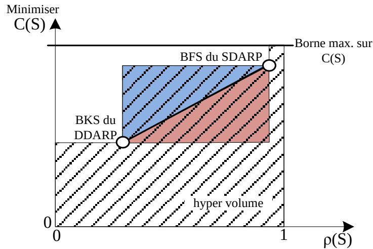
Figure 4.45 : Borne supérieure à l'hypervolume
