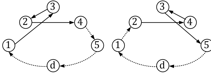
Figure 2.62 : Deux autres mouvements explorés dans le bloc r\text{-}4\text{opt}^*
