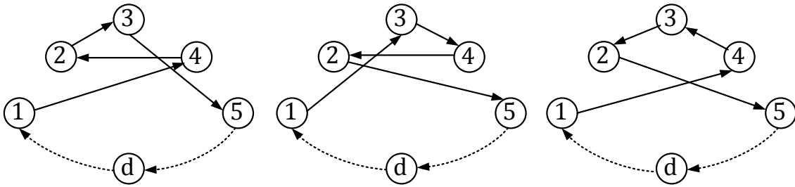
Figure 2.61 : Les trois mouvements du bloc r\text{-}4\text{opt}^* dans une tournée
