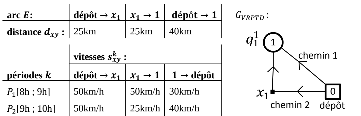
Figure 3.7 : Un exemple de pour le calcul d'un chemin
