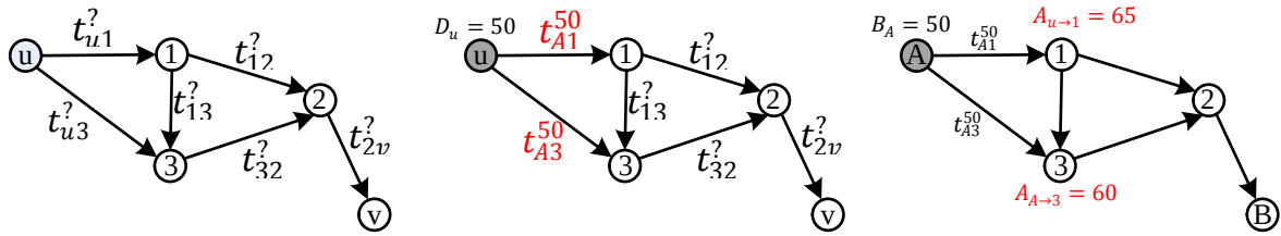
Figure 3.17 : Graphe initial, date de départ de u fixée, propagation des dates d'arrivée sur \delta^+ de u (1 et 3)
