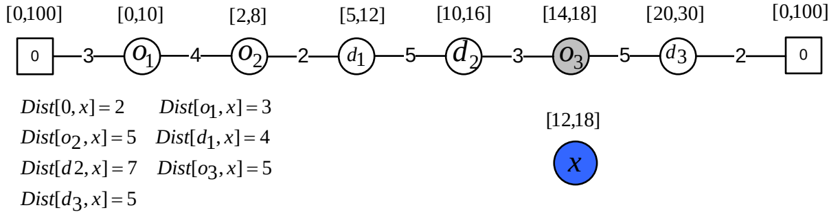
Figure 20 : La borne supérieure d'insertion pour un sommet x
