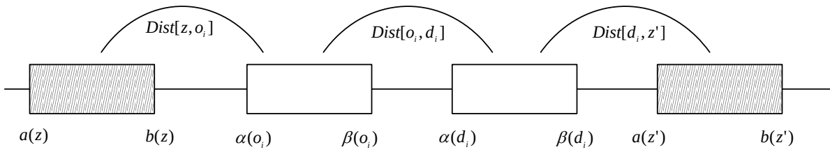
Figure 23 : Illustration pour EC2
